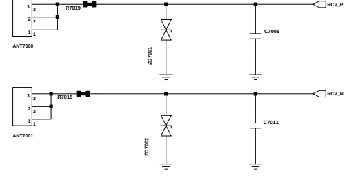
RCV CONTACT
